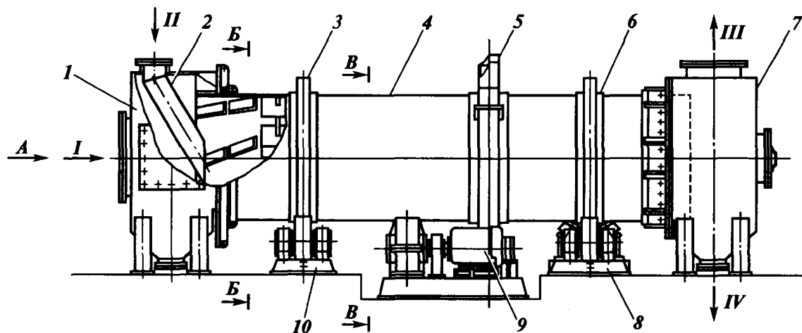
Рис. X-14. Барабанная сушилка:
